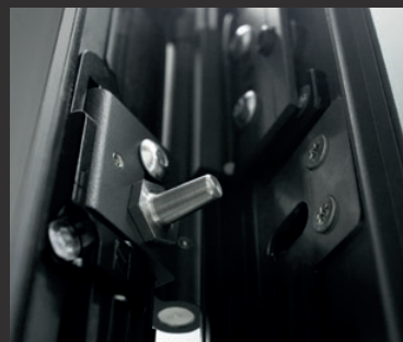
Антизломні штирі - це додаткове устаткування, яке покращує антизломні характеристики дверей. Вони встановлюються з боку петель на дверному полотні та на коробці. Залежно від необхідного ступеню безпеки можна застосовувати різну кількість наборів для одного полотна.
